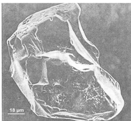
Ryc. 26. Nieregularne zarysy, ślady rozpuszczania i wytrącania krzemionki. Ziarno transportowane w lodowcu i przez wodę.
