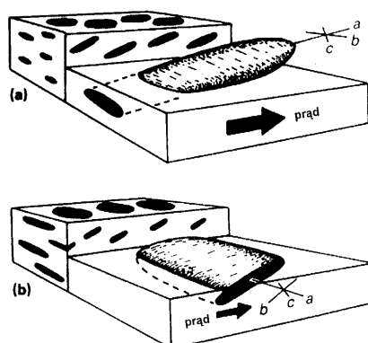
Ryc. 65. Imbrykacja otoczków: (a) osie najdłuższe - a - równoległe do kierunku prądu; (b) osie najdłuższe prostopadłe do kierunku prądu (z Lindholm 1987)
