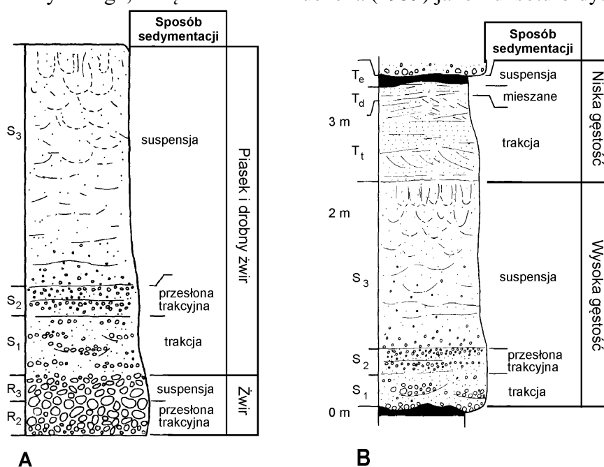
Ryc. 110. Profile ławic idealnych osadów prądów zawiesinowych o wysokiej gęstości (według Lowe 1982). A - profil ławicy prądu żwirowo-piaszczystego (Sekwencja R_1 - S_3 = sekwencja Lowe'a ); B - profil ławicy prądu piaszczystego
