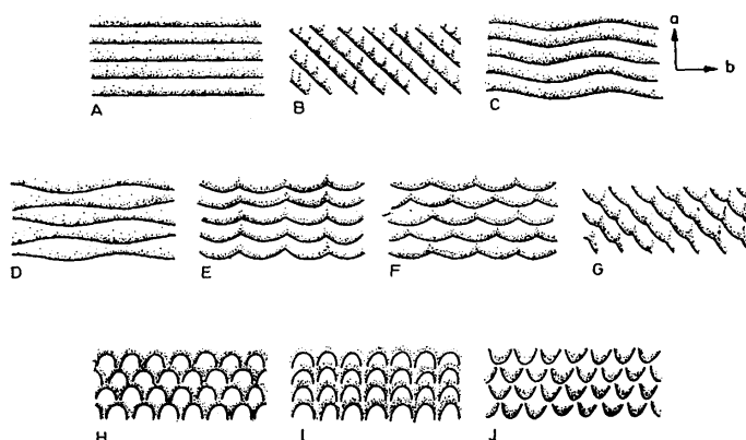
Ryc. 50. Zróżnicowanie zmarszczek w planie (z Gradziński et al. 1986)
