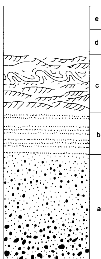
Ryc. 104. Profil ławicy zawiesinowca (turbidyty) z sekwencją Boumy (pionowa sekwencja członów teksturowo-strukturalnych, Bouma 1962)
