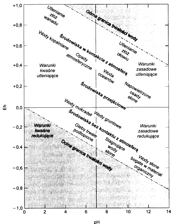
Ryc. 140. Eh i pH wód w różnych środowiskach (według Baas Becking et al. 1964)
