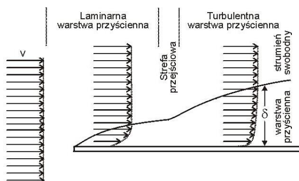
Ryc. 37. Rozwój laminarnej i turbulენტnej warstwy przyściennej (z Gradziński et al. 1986)
