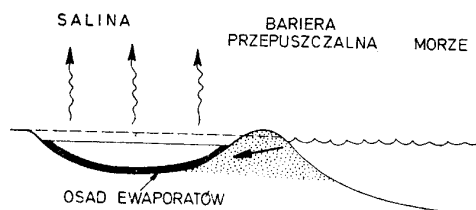
Ryc. 144. Sedymentacja ewaporatów w salinie, słonej zatoce z przesiąkaniem solanki przez barierę. Osad bariery w strefie odpływu solanki może ulegać dolomityzacji (por. model formowania dolomitów).
