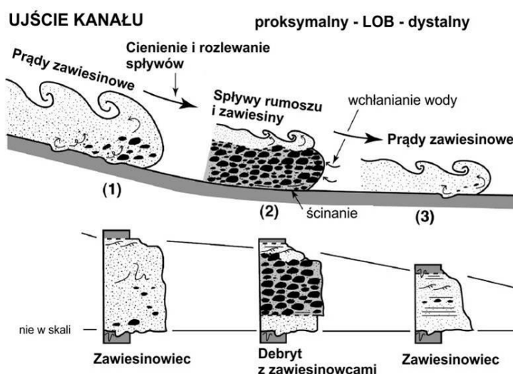
Ryc. 117. Formowanie kogenetycznego turbidytu-debrytu (debrytu powiązanego; według Ito 2008)
