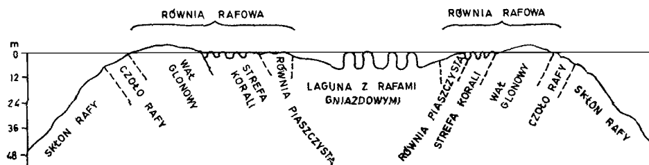
Ryc. 154. Przekrój morfologiczny przez rafę barierową (Maxwell 1968, z: Gradziński et al. 1986)
