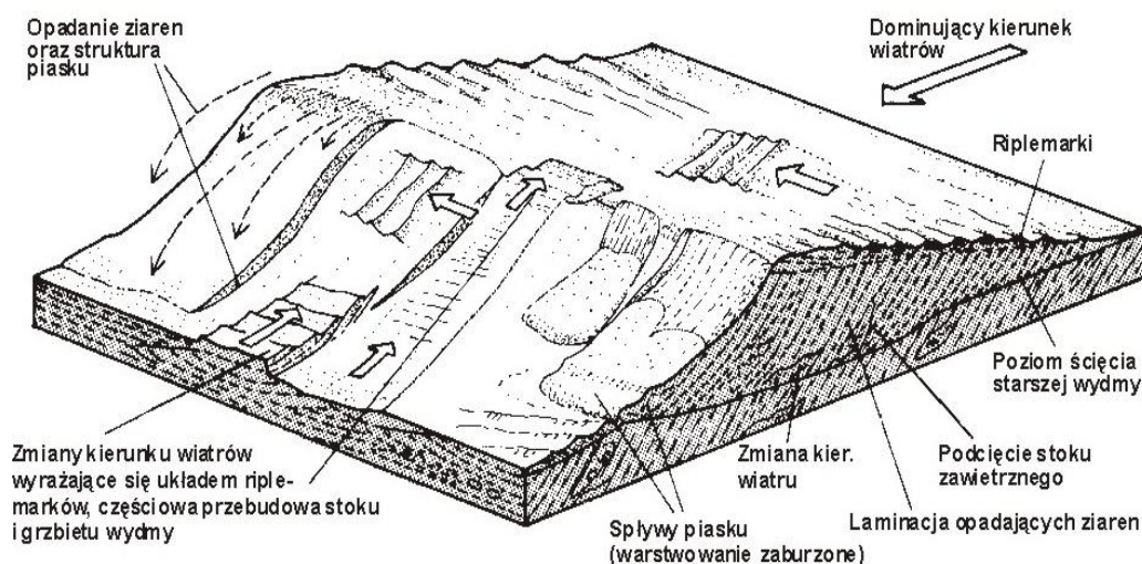
Ryc. 100. Duża wydma poprzeczna z jednokierunkową laminacją przekatną, z nałożonymi riplemarkami formowanymi przez wiatry wiejące z różnych kierunków (według Einsele 1992)
