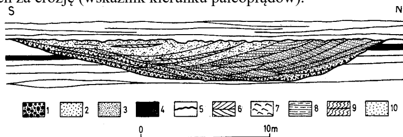
Ryc. 86. Poprzeczny przekrój przez kanał erozyjny (według Gradziński 1970). 1 – zlepienie śródformacyjny, 2 – piaskowiec, 3 – mułowiec, 4 – iłowiec z konglomeratami, 5 – powierzchnia erozyjna, 6 – warstwowanie przekątne o dużej skali, 7 – warstwowanie przekątne o małej skali, 8 – laminacja pozioma, 9 – zaburzone warstwowanie przekątne, 10 – piaskowiec masywny
