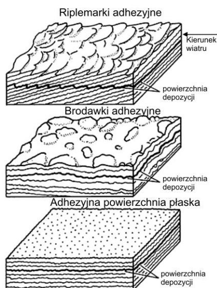
Ryc. 98. Struktury piasku eolicznego kształtowane przez adhezję (wg Kocurek & Fielder, 1982)
