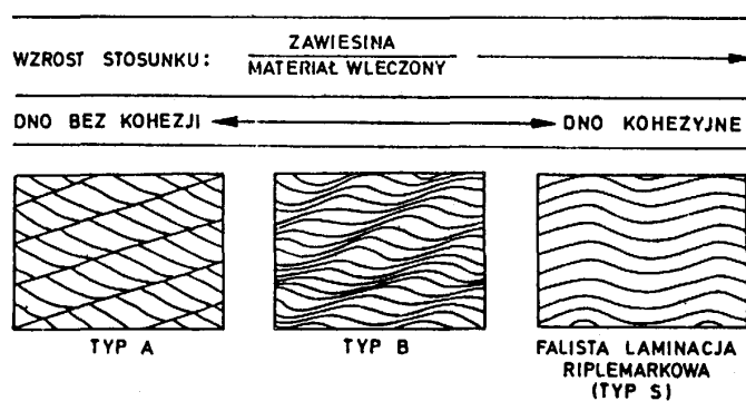
Ryc. 59. Główne typy struktur riplemarków wstępujących (z Gradziński et al. 1986)
