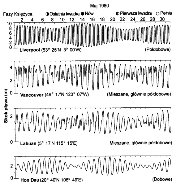
Ryc. 81. Krzywe pływów w maju 1980 r. ukazujące częstotliwości półdobowe i dobowe (Admiralty Time Tables; Allen 2001)
