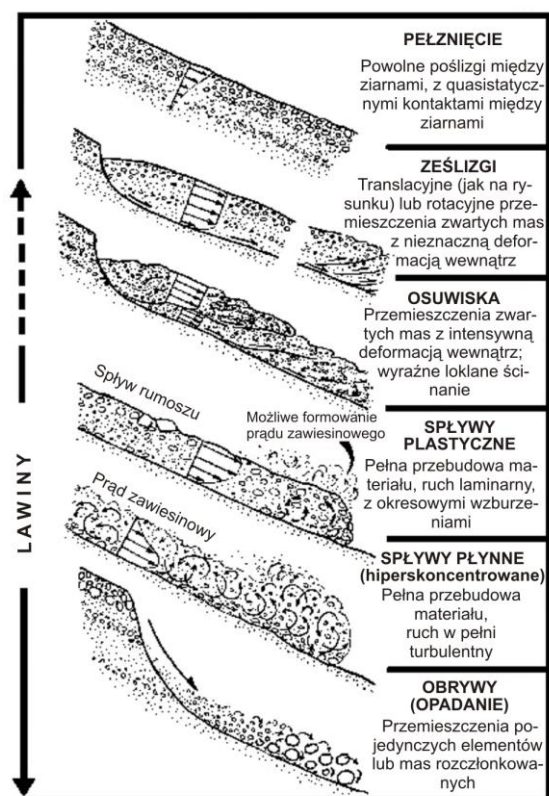
Rys. 119. Podstawowe rodzaje napowietrznych grawitacyjnych procesów sedymentacyjnych zależnie od własności reologicznych przemieszczanej materii i tempa przebiegu procesu, według W. Nemeč, materiały niepublikowane
