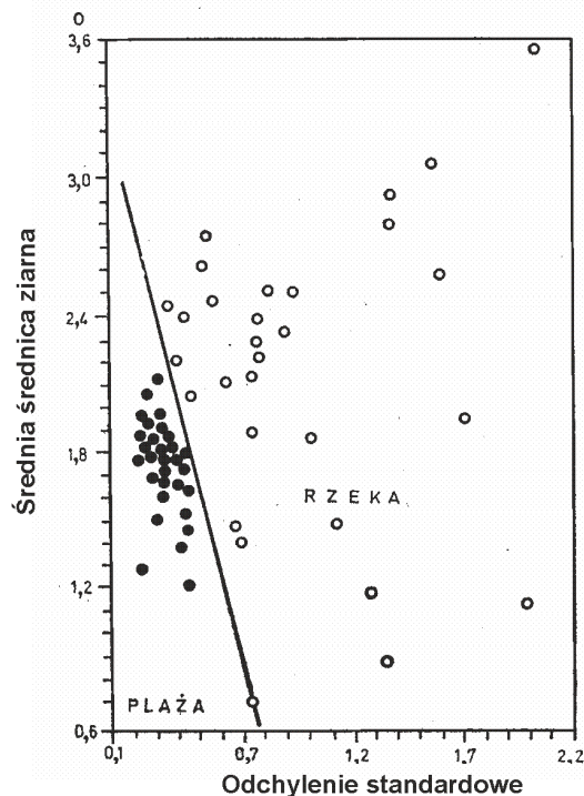
Ryc. 18. Zależność między standardowym odchyleniem a średnicą ziarna dla piasków plażowych i rzecznych (według Moiola & Weiser 1968)
