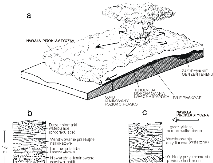
Ryc. 126. Nawała piroklastyczna i jej osady (według Einsele 1992)
