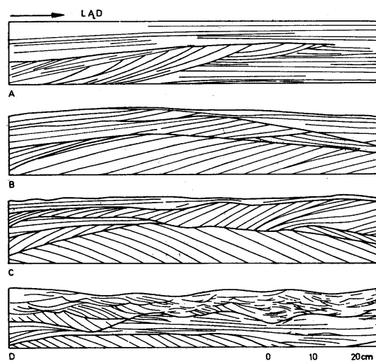
Ryc. 75. Struktury osadów litoralnych na wybrzeżach bezrewowych (wg Clifton et al. 1971). A - zmywu, B - strefa przyboju, C - strefa wzrostu fali bliższa brzegu, D - strefa wzrostu fali część dalsza
