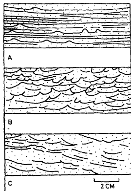
Ryc. 137. Różne typy struktur miseczkowych (wg Gradziński et al. 1986)
