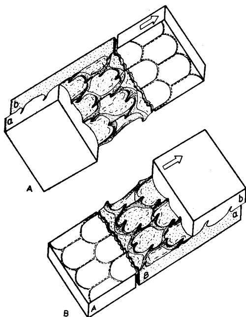
Ryc. 129. Wpływ naprężeń ścinających na kolumny diapirowi (według Anketell et al., 1970; z: Gradziński et al. , 1986)
