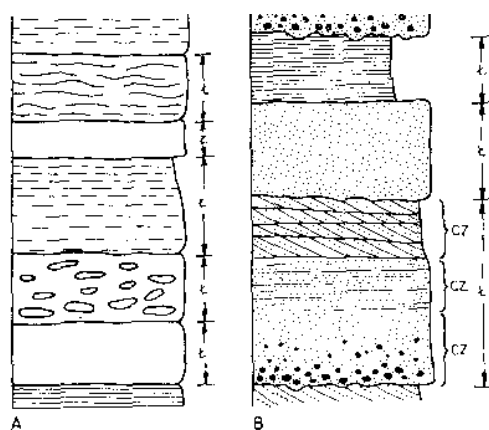
Ryc. 3. Ławice: A – przykład z serii wapiennej, B – przykład z utworów fliszowych. L – ławica, CZ – człon ławicy (z Gradziński et al. 1986)
