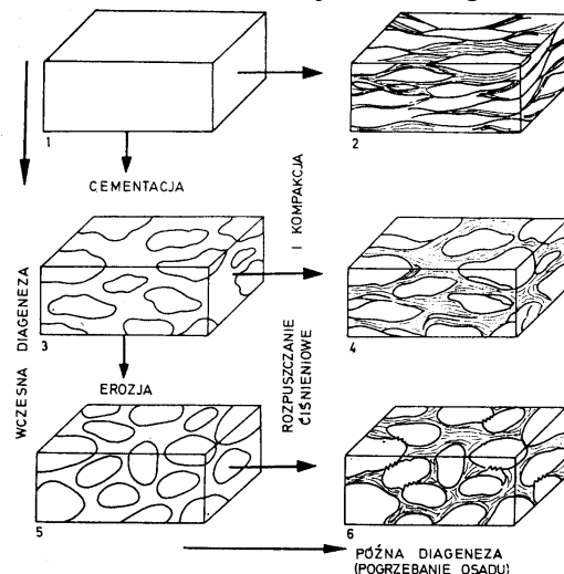
Ryc. 136. Formowanie struktur gruzłowych według Gradziński et al. 1986
