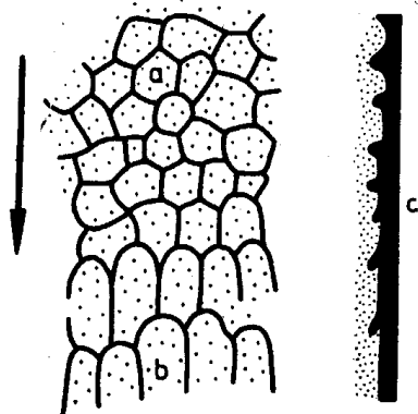
Ryc. 132. Przechodzenie struktur wielobocznych w struktury łuskowe (według Dżułyński & Simpson, 1966)
