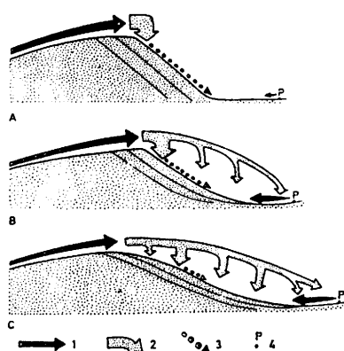
Ryc. 54. Kształt stoku zaprawdowego nierówności dna, w tym riplemarków w zależności od natężenia transportu trakcyjnego (A – najniższe, C – najwyższe) (z Gradziński et al. 1986)
