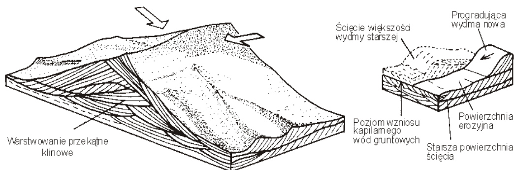
Ryc. 100. Duża wydma poprzeczna z jednokierunkową laminacją przekatną, z nałożonymi riplemarkami formowanymi przez wiatry wiejące z różnych kierunków (według Einsele 1992)
