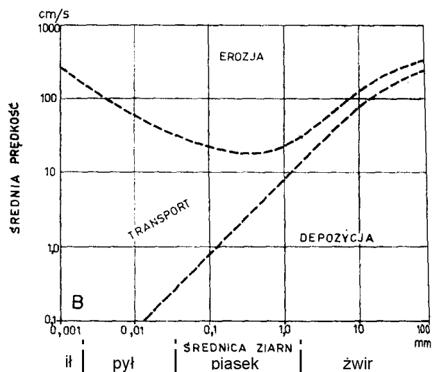
Ryc. 46. Empiryczna zależność erozji, transportu i depozycji dla ziaren różnej wielkości od średniej prędkości przepływu prądu (według Hjulstrom 1935 z: Gradziński et al. 1986)
