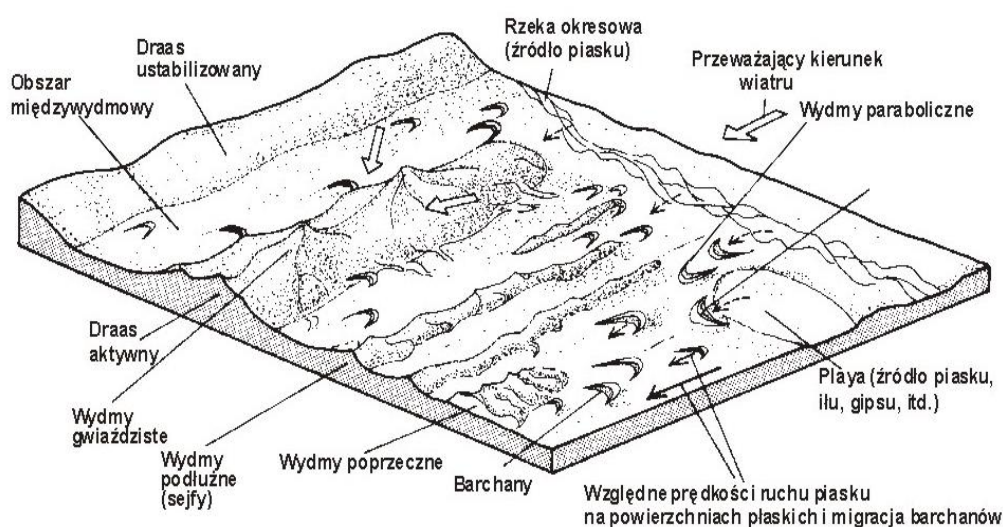
Ryc. 99. Główne rodzaje wydm w odniesieniu do przeważającego kierunku wiatrów. Od prawej do lewej wzrost dostawy i tempa akumulacji piasku oraz prędkości migracji wydm (wg Einsele, 1992)
