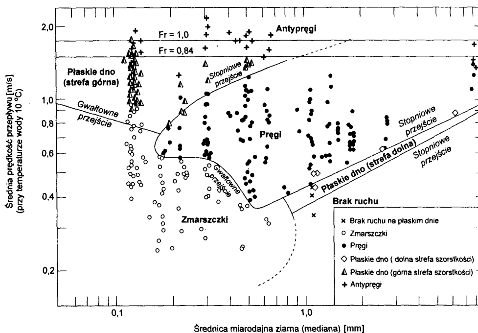
Ryc. 51. Formy dna a mediana ziarna pokrywającego dno i średnia prędkość przepływu (z Allen 2001)
