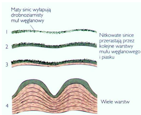
Ryc. 160. Rozwój stromatolitów – efekt biernego wychwytywania i wiązania cząstek osadu przez sinice
