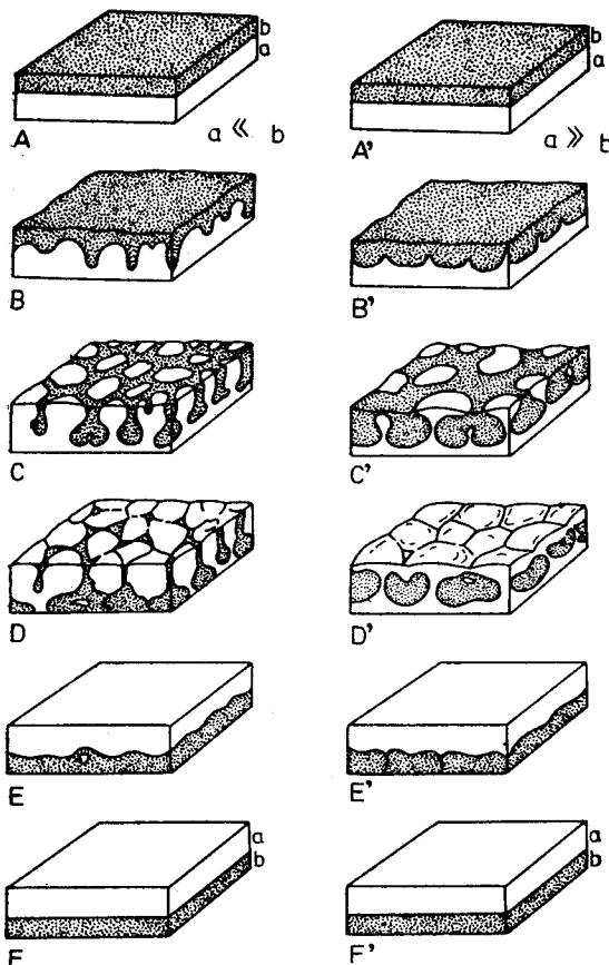
Ryc. 128. Kolejne stadia rozwojowe struktur deformacyjnych w układach nieruchomych według Cegła & Dżułyński, 1970)
