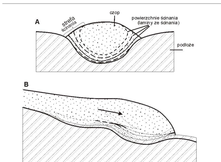
Ryc. 40. Struktura czoła zamierającego spływu płynu nienewtonowskiego; A – przekrój prostopadły do kierunku spływu, B – przekrój równoległy do kierunku spływu
