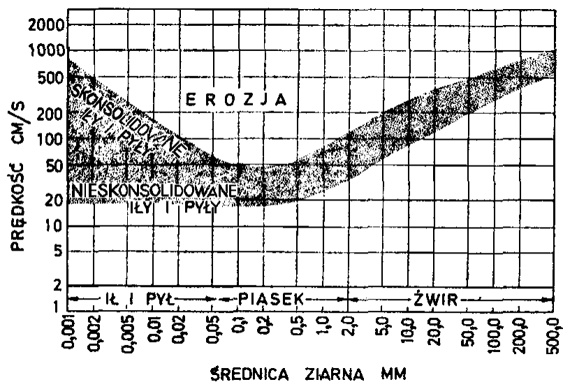
Ryc. 47. Diagram Hjulstroma w wersji zmodyfikowanej przez Sundborga (1956) (z: Gradziński et al. 1986)
