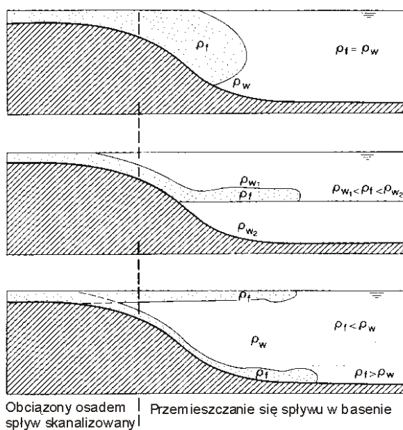
Ryc. 118. Rodzaje spływów gęstościowych zależnie od relacji gęstości spływu do gęstości otaczającej wody (zmodyfikowane z Bates, 1953 przez Muldera i In., 1997)
