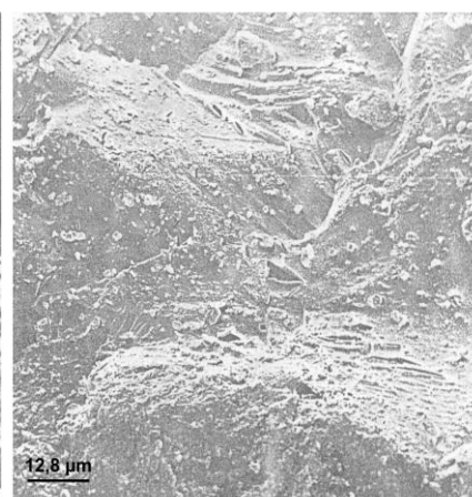
Ryc. 29. Struktury rozkładu powierzchni ziarna nałożone na wylomy muszlowe. Osady współczesne, Uganda.
