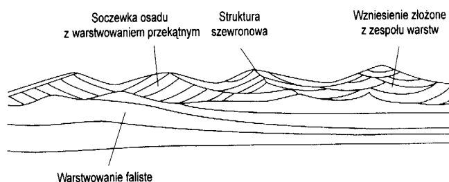
Ryc. 74. Struktura osadu tworzącego riplemarki falowe (z Allen 2001)
