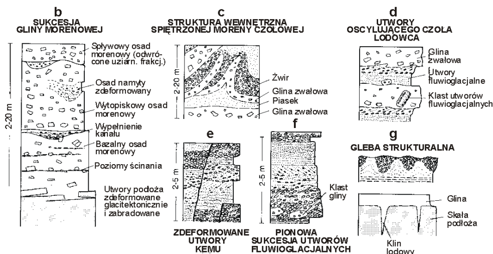
Ryc. 102. Procesy sedymentacyjne związane z lodowcami kontynentalnymi i ich produkty, (według Einsele 1992). A – Procesy sedymentacyjne i formy akumulacji osadu u czoła wycofującego się lodowca; B - Osady polodowcowe wytopiskowe i wodnolodowcowe
