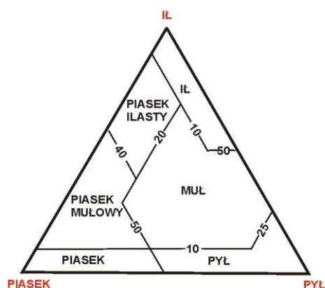
Ryc. 21. Nazwy osadów złożonych z materiału piaszczystego, pyłowego i łuowego (według: Shepard, 1954)
