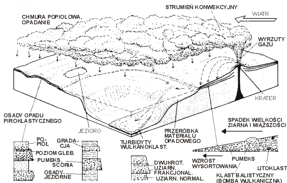
Ryc. 122. Erupcja pliniańska i jej produkty (według Einsele 1992)
