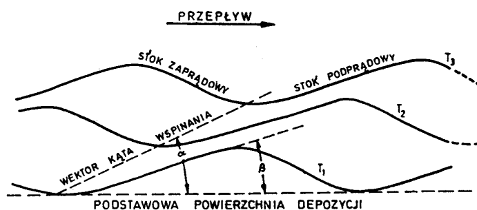
Ryc. 58. Migracja riplemarków w warunkach agradacji (z Gradziński et al. 1986)
