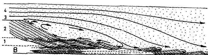
Ryc. 53. Kształtowanie sedimentacji na stoku zaprawdowym i przedpolu riplemarka dużego (pręgi) (z Gradziński et al. 1986)
