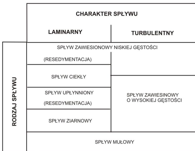
Ryc. 107. Klasyfikacja podwodnych grawitacyjnych spływów osadu zależnie od sposobu ruchu spływu (według Lowe 1982)
