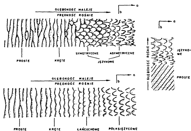
Ryc. 55. Kształt riplemarków w planie w zależności od głębokości i prędkości prądu (z Gradziński et al. 1986)
