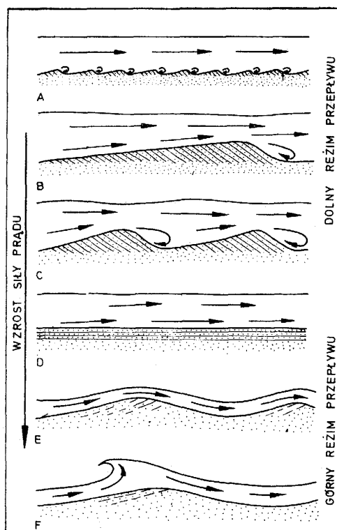
Ryc. 57. Formy dna i struktura budującego je osadu (z Gradziński et al. 1986)
