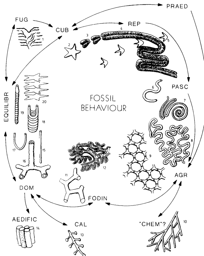
Ryc. 164. Etologiczna klasyfikacja struktur bioturbacyjnych (skamieniałości śladowych) według Bromley 1996.
