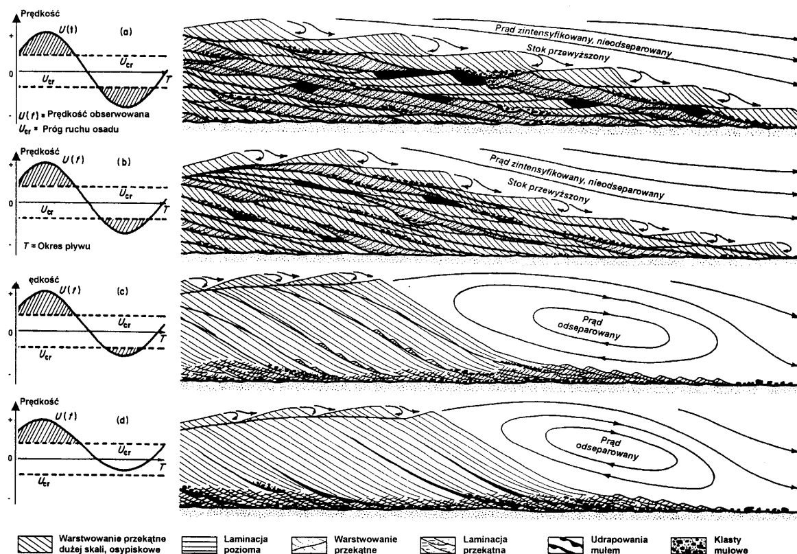
Ryc. 82. Modele struktury wewnętrznej pływowych fal piaskowych kontrolowanej relacją prędkości prądu przyływu do prądu odpływu. W modelach pokazana jest część fali piaskowej zwrócona w kierunku dominującego prądu. W modelach a i b stoki fal oraz miąższości zestawów lamin formowanych w efekcie jednej fazy pływu są nieco przewyższone. Zestawy wstępującej laminacji przekątnej w modelach a i b są formowane kiedy na fali piaskowej tworzą się riplemarki prądowe małej skali. Riplemarki duże tworzą zestawy warstwowania przekątnego jodełkowego. Fale w modelach a i b mają charakter grzbietów wydłużonych zgodnie z kierunkiem prądów zaś w modelach c i d rozciągają się prostopadłe do kierunku prądów (wg Allen 1984)
