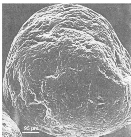
Ryc. 28. Ziarno zaokrąglone, pokryte pochylonymi płytkami i dużymi zagłębieniami V-kształtnymi. Ziarno transportowane przez wiatr. Sahara, plejstocen
