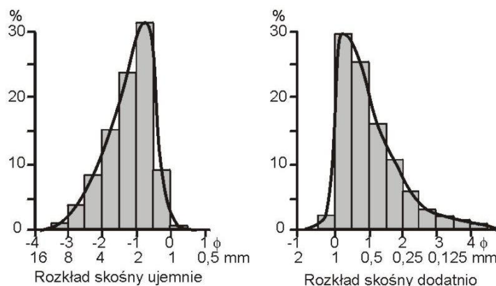
Ryc. 16. Asymetria rozkładów uziarnienia
