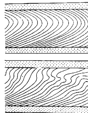
Ryc. 135. Deformacyjne fałdy obalone (według Allen & Banks, 1972, z: Gradziński et al., 1986)
