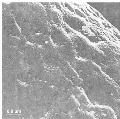
Ryc. 25. Struktury z rozpuszczania i pochylone płytki. Fragment powierzchni ziarna z ryciny obok.
