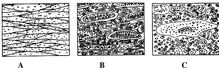
Ryc. 124. Najważniejsze rodzaje skał piroklastycznych ze szlaką (według Fuechtbauer 1988). A – aglutynat, B – aglomerat, C – brekcja wulkaniczna
