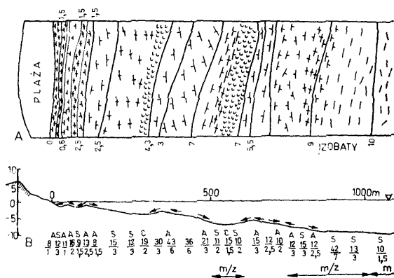
Ryc. 72. Formy dna i kierunki transportu osady w strefie przybrzeżnej morza (Litoralnej) na planie (A) i w przekroju (B) (wg Rudowski, 1970). A - asymetryczne, S - riplemarki symetryczne, C - riplemarki językowe, m/z - muł w brzdach riplemarków, m - muł na dnie, 12/3 - rozstęp riplemarków
