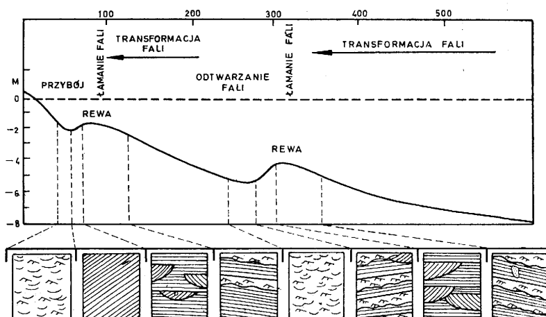
Ryc. 76. Struktury osadów litoralnych na wybrzeżach rewowych (wg Davidson-Arnott & Greenwood 1976).
