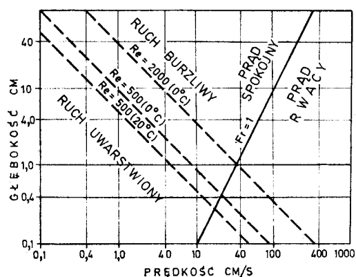
Ryc. 35. Typ przepływu a głębokość i prędkość strumienia (z Gradziński et al. 1986)
