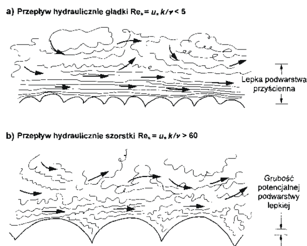
Ryc. 39. Przepływ hydraulicznie gładki lub szorstki, w zależności od liczby Reynoldsa obliczonej dla powierzchni ścianki u_* k / \nu
