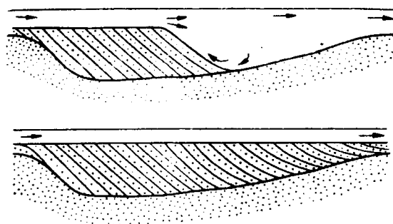
Ryc. 64. Wpływ spłykania się zagłębienia dna na kształt zarysu lamin przekątnych w przekroju równoległym do kierunku przepływu prądu zasypującego zagłębienie (z Gradziński et al. 1975)
