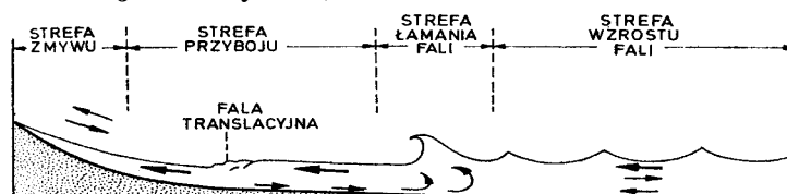
Ryc. 70. Strefy transformacji fali (wg Ingle 1966)
