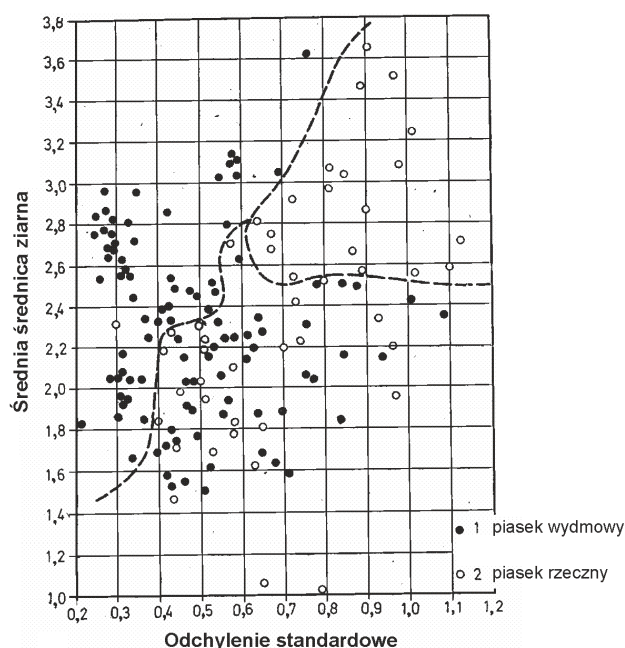
Ryc. 19. Zależność między standardowym odchyleniem a średnicą ziarna dla piasków wydymowych i rzecznych (według Friedman 1961)
