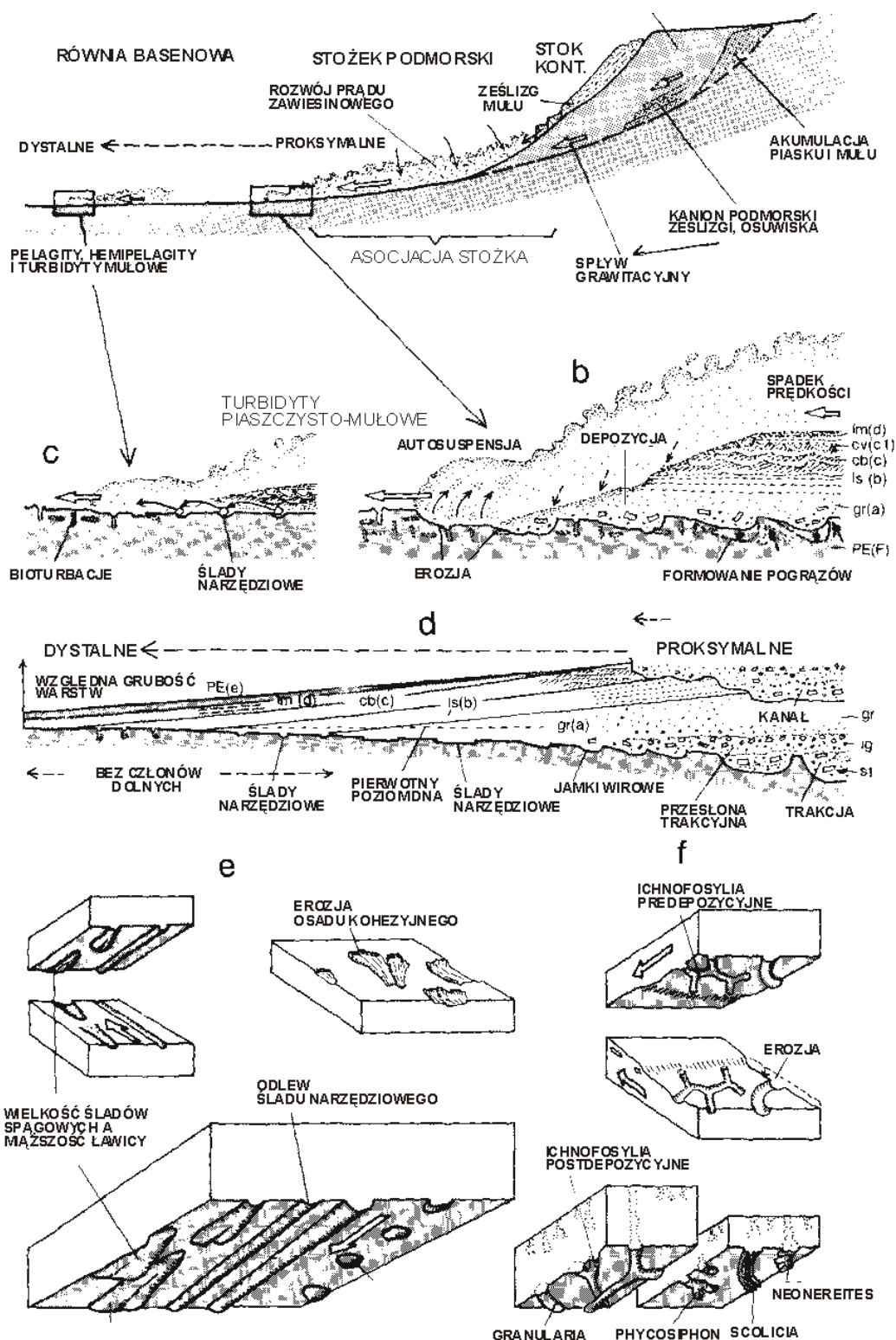
Ryc. 114. Model koncepcyjny formowania zawiesinowców piaszczystych (turbidytów) proksymalnych i dystalnych oraz struktury wewnętrzne takich utworów. a – przechodzenie osuwania stoku basenowego (osuwisko, spływ mułowy, spływ rumoszywy kohezyjny, kolizyjny) w spływ zawiesinowy (prąd zawiesinowy); b – zawiesinowiec z pełną sekwencją strukturalnych członów sekwencji Boumy (w nawiasach), ze zmodyfikowanymi symbolami opisu oraz autosuspensja napędzana przez turbulencje; c – zawiesinowiec bardziej dystalny bez erozji i dolnych członów sekwencji Boumy; d – wyidealizowane następstwo osadów deponowanych ze spływu zawiesinowego; e – geneza różnych rodzajów hieroglify (według Einsele 1992)
