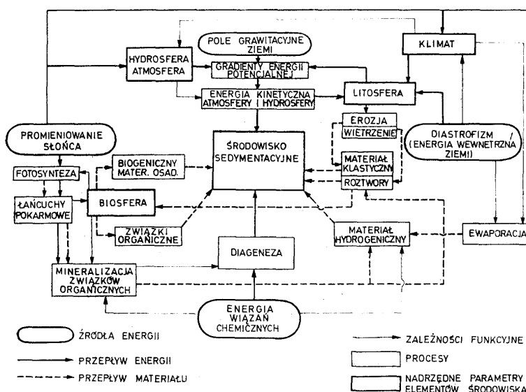
Ryc. 5. Źródła energii a procesy sedimentacyjne – model zależności (wg Gradziński et al. 1986)
