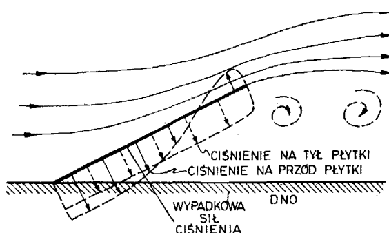
Ryc. 44. Wzór przepływu i hipotetyczny rozkład ciśnień wokół płytki pochylonej zapadem pod prąd (zimbrykowanej) przy umiarkowanie dużej wartości liczby Reynoldsa (według Middleton & Southard 1978, zmodyfikowane przez Gradziński et al. 1986)
