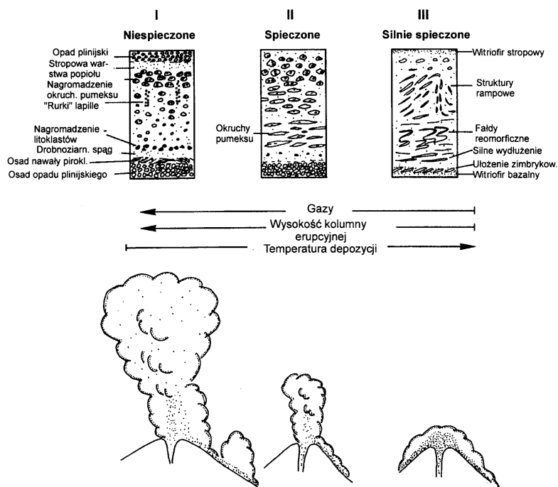
Ryc. 125. Charakter erupcji a rodzaj i cechy ignimbrytu według Fuechtbauer 1988
