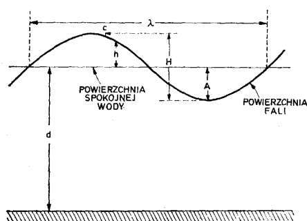
Ryc. 68. Parametry fali postępującej A – amplituda; d – głębokość zbiornika, \lambda – długość fali; H – wysokość fali
