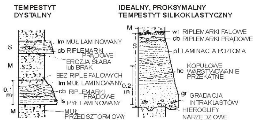
Ryc. 79. Profile modelowe tempeptytów silikoklastycznych (wg Einsele 1992)
