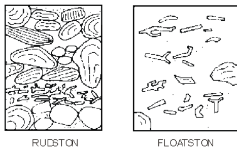
Ryc. 155. Podstawowe rodzaje wapieni formowane w obrębie nasypu u podnóża raf (talusa)
