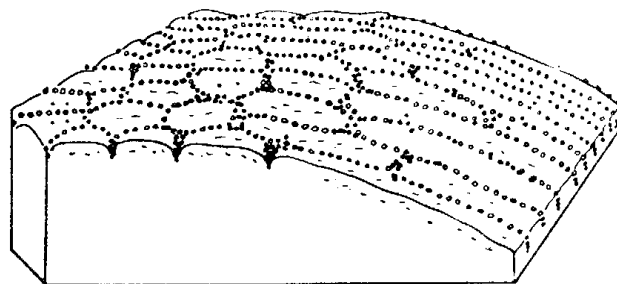
Ryc. 131. Gleby strukturalne według Sharpe'a (1938). Sieć kamienista przechodzi w obrebie stoku w pasy kamieniste
