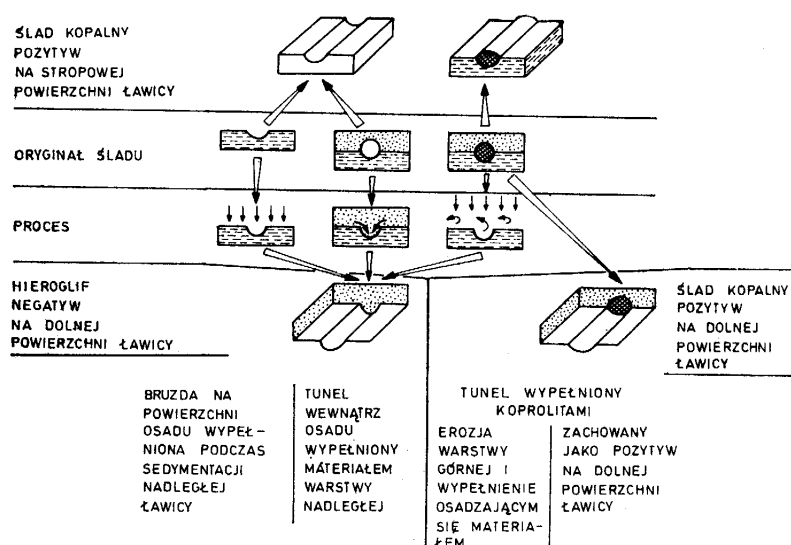
Ryc. 163. Sposoby fosylizacji ich noskamieniałości (z Gradziński et al. 1986)
