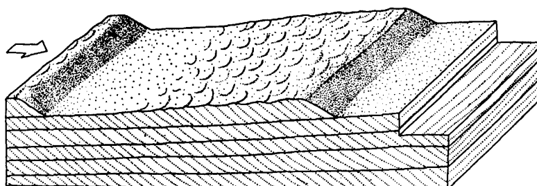
Ryc. 61. Struktura osadu formowanego poprzez sedymentację na falach piaskowych (warstwowanie przekątne tabularne) (z Gradziński et al 1986)
