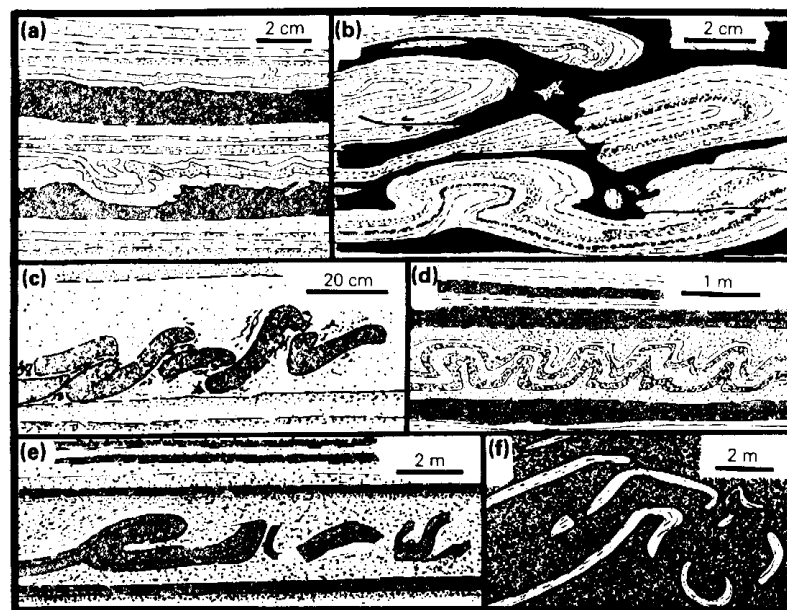
Ryc. 133. Fałdy i płyty deformacyjne, uławicenie zaburzone
