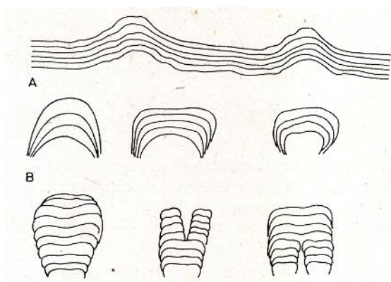
Ryc. 161. Najprostsze rodzaje stromatolitów. A – laminy ciągłe, kopułkowato wygięte, B – formy kopułkowate, laminy nieciągłe, C – formy kolumnkowe, laminy nieciągłe (z Gradziński et al. 1986).
