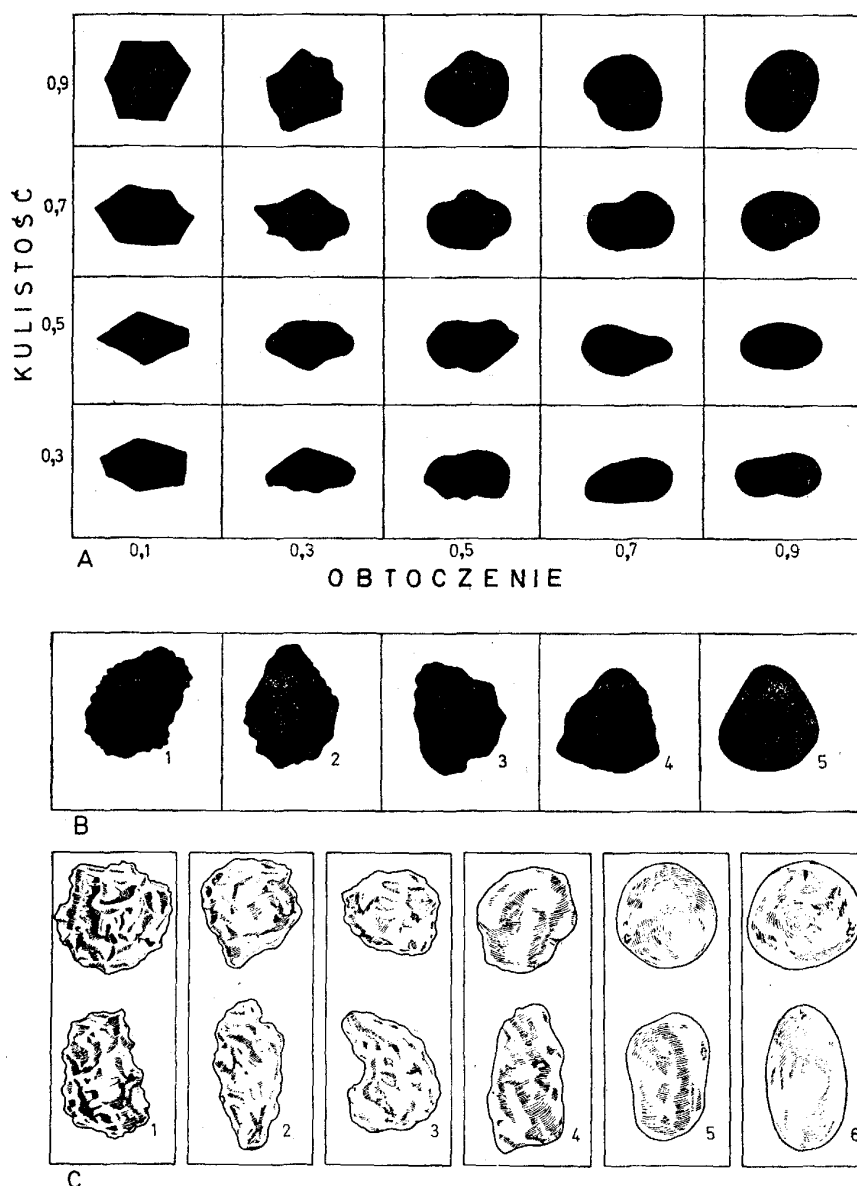
Ryc. 23. Wzorce do wizualnego określania stopnia obtoczenia z Gradziński et al. , 1986. A — wzorec według Krumbeina i Slossa (1963): wyróżnione cztery klasy kulistości i pięć klas obtoczenia; podane wartości liczbowe kulistości i obtoczenia; B — wzorec według Petijohna (1975): klasy stopnia obtoczenia nierównej szerokości; szerokość klasy rośnie ze wzrostem stopnia obtoczenia ziarna; ziarna: 1 — ostrokrawędziste, 2 — półostrokrawędziste, 3 — półobtoczzone, 4 — obtoczzone, 5 — dobrze obtoczzone; C — wzorec według Powersa (1953): klasy stopnia obtoczenia nierównej szerokości; górny rząd: ziarna o kształcie kulistym, dolny rząd — ziarna wydłużone; ziarna: 1 — bardzo ostrokrawędziste, 2 — ostrokrawędziste, 3 — półostrokrawędziste, 4 — półobtoczzone, 5 — obtoczzone, 6 — dobrze obtoczzone.
