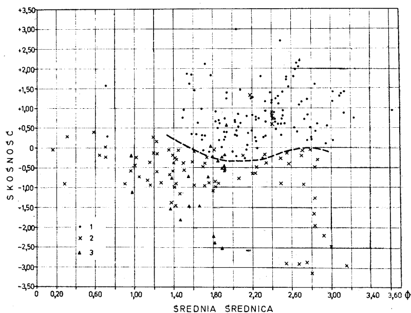
Ryc. 17. Zależności między skośnością a średnią średnicą ziarna piasku wydmowego i plażowego (według Friedman, 1961). 1 — piasek wydmowy, 2 — piasek z plaży na wybrzeżu oceanu, 3 — piasek z plaży na wybrzeżu jeziora
