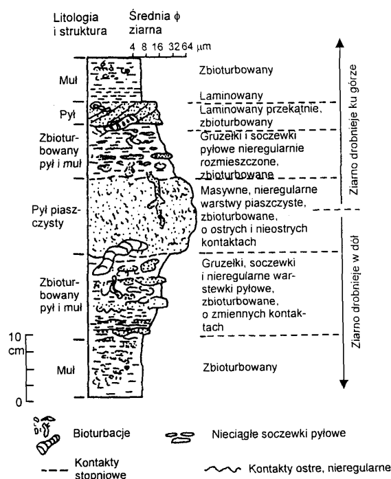
Ryc. 85. Modelowy profil konturytów (według Stow et al. 1986)
