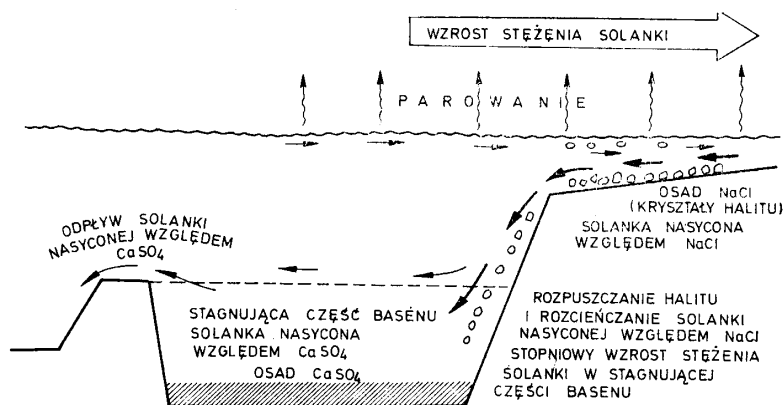
Ryc. 150. Sedymentacja ewaporatów w basenie głębokim z odpływem solanki. Faza trwałej akumulacji \text{CaSO}_4 i czasowego wytrącania \text{NaCl} , który ulega rozpuszczeniu w stagnującej części basenu, zwiększając w niej stężenie solanki. Po osiągnięciu nasylenia względem \text{NaCl} w stagnującej części basenu rozpoczyna się trwała akumulacja halitu (wg Schmalz, 1969 zmienione przez Gradziński et al., 1986)
