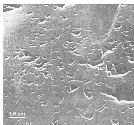
Ryc. 27. Bruzdy i V-kształtne wylomy produkowane przy transporcie ziarna przez wodę. Szelf, Argentyna, plejstocen
