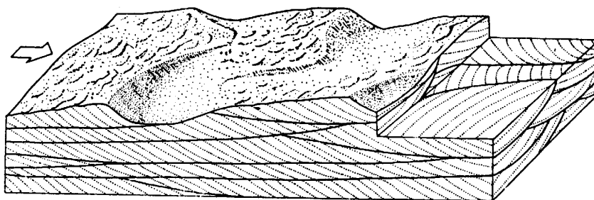
Ryc. 62. Struktura osadu formowanego poprzez sedymentację na dużych riplemarkach krętożrbietowych, językowych, półksiężycowych (warstwowanie przekątne rynnowe) (z: Gradziński et al. 1986)
