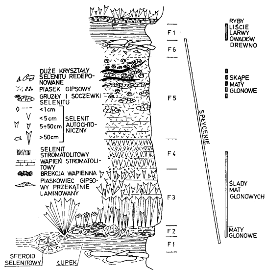
Ryc. 151. Pełny cykl sedymentacyjny gipsów złożony z sekwencji sześciu facji (F1-F6) (według Ricci-Lucchi 1976)
