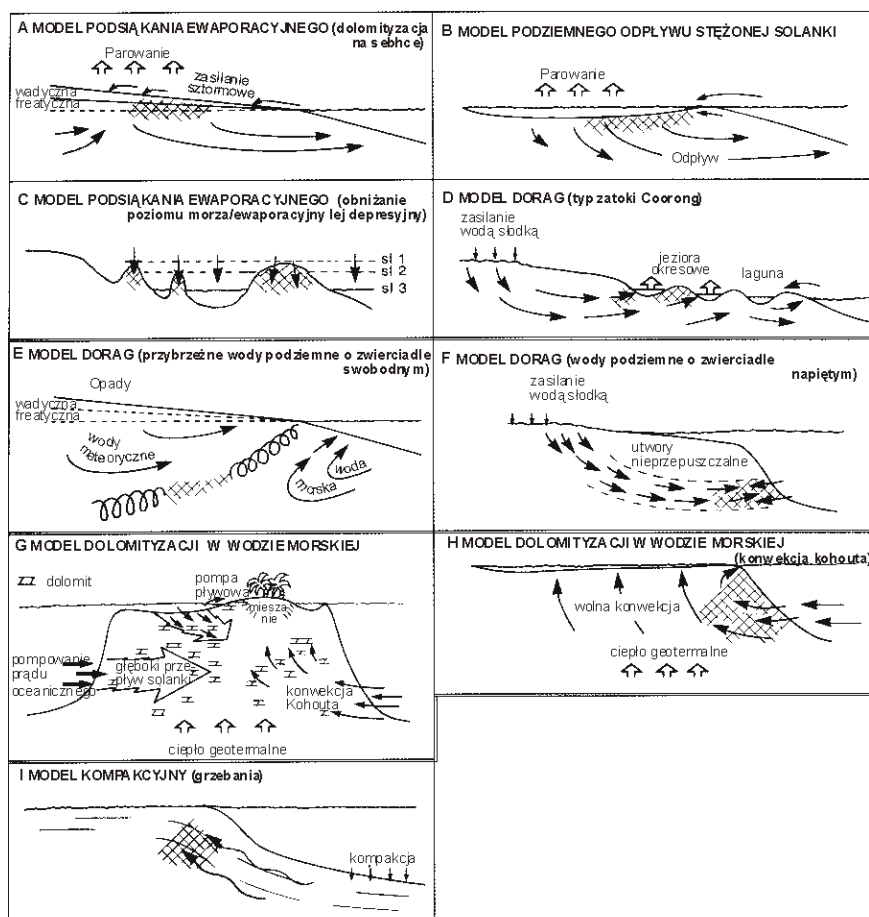
Ryc. 143. Modele formowania dolomitów (z Fluegel 2003).
