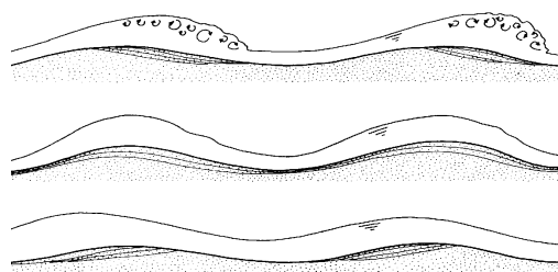
Ryc. 56. Formowanie i struktura wewnętrzna antydiun (antypręgi) (z Allen 2001)
