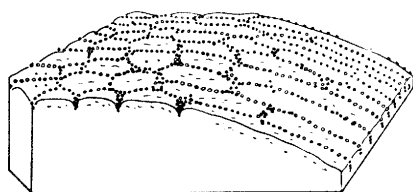
Ryc. 120. Gleby strukturalne widok na powierzchni i w przekroju, według Sharpe'a (1938). Sieć kamienista przechodzi w obrębie stoku w pasy kamieniste
