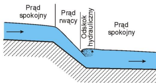
Ryc. 34. Zapis przechodzenia między prądem spokojnym i rwącym
