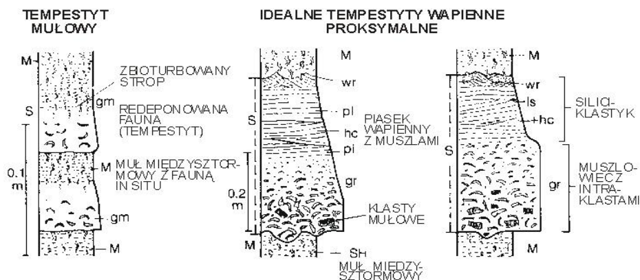
Ryc. 78. Profile modelowe tempeptytów wapiennych (wg Einsele 1992)
