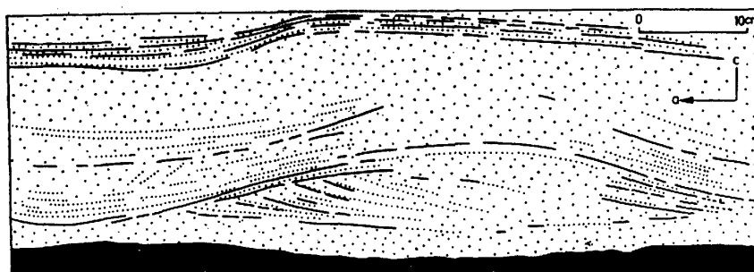
Ryc. 63. Struktura osadu deponowanego na antypęgach (antydiunach; z Gradziński et al. 1986)
