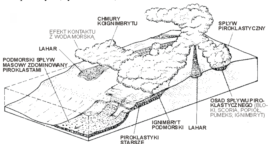
Ryc. 123. Załamanie kolumny erupcyjnej i formowanie spływów piroklastycznych (ignimbrytowych; według Einsele 1992)
