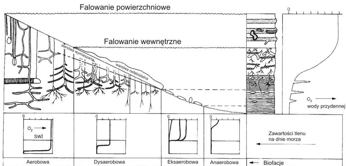
Ryc. 167. Zawartość tlenu na dnie morza a ukształtowanie (głębokość i charakter) bioturbacji (według Savrda et al. 1991)
