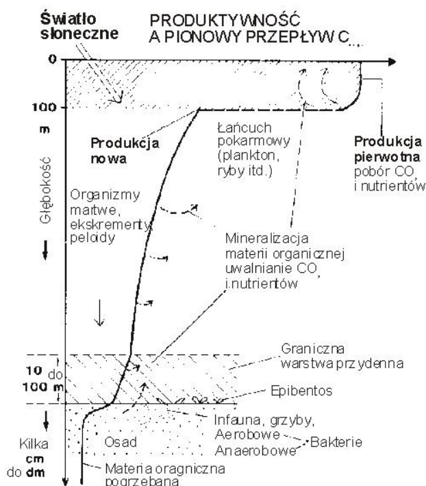
Ryc. 157. Procesy kontrolujące pionowy przepływ węgla organicznego ze strefy produkcji pierwotnej po grzebanie na dnie morza według Einsele 1992
