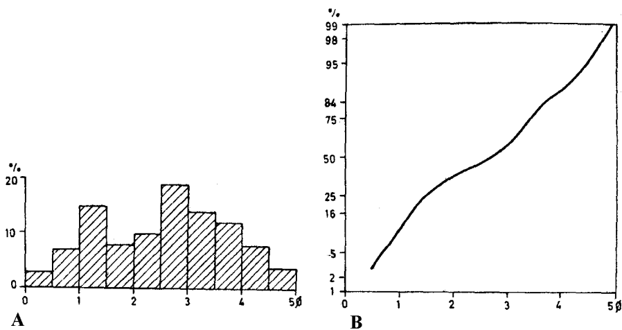
Ryc. 15. Rozkład bimodalny, A - histogram, B - krzywa kumulacyjna
