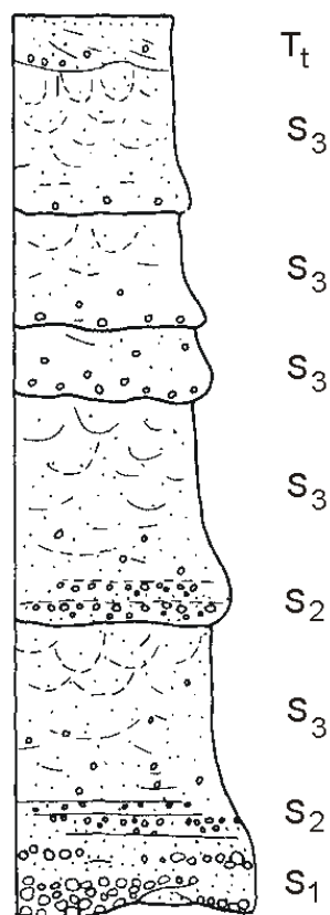
Ryc. 111. Model ławicy osadzonej z wielopulsowego piaszczystego prądu zawiesinowego o wysokiej gęstości (według Lowe 1982)
