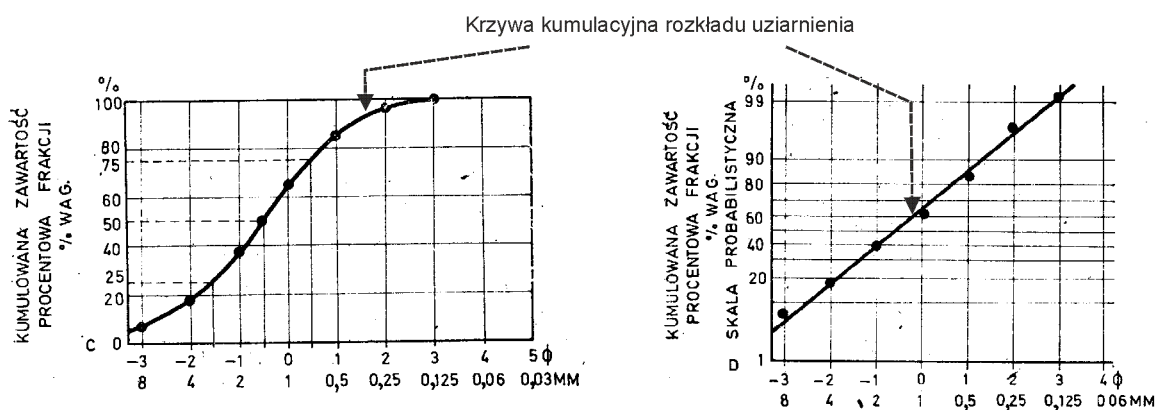
Ryc. 14. Krzywe kumulacyjne rozkładu uziarnienia na siatce ze skalą arytmetyczną (C) i siatce ze skalą prawdopodobieństwa (według Gradziński et al. 1986)
