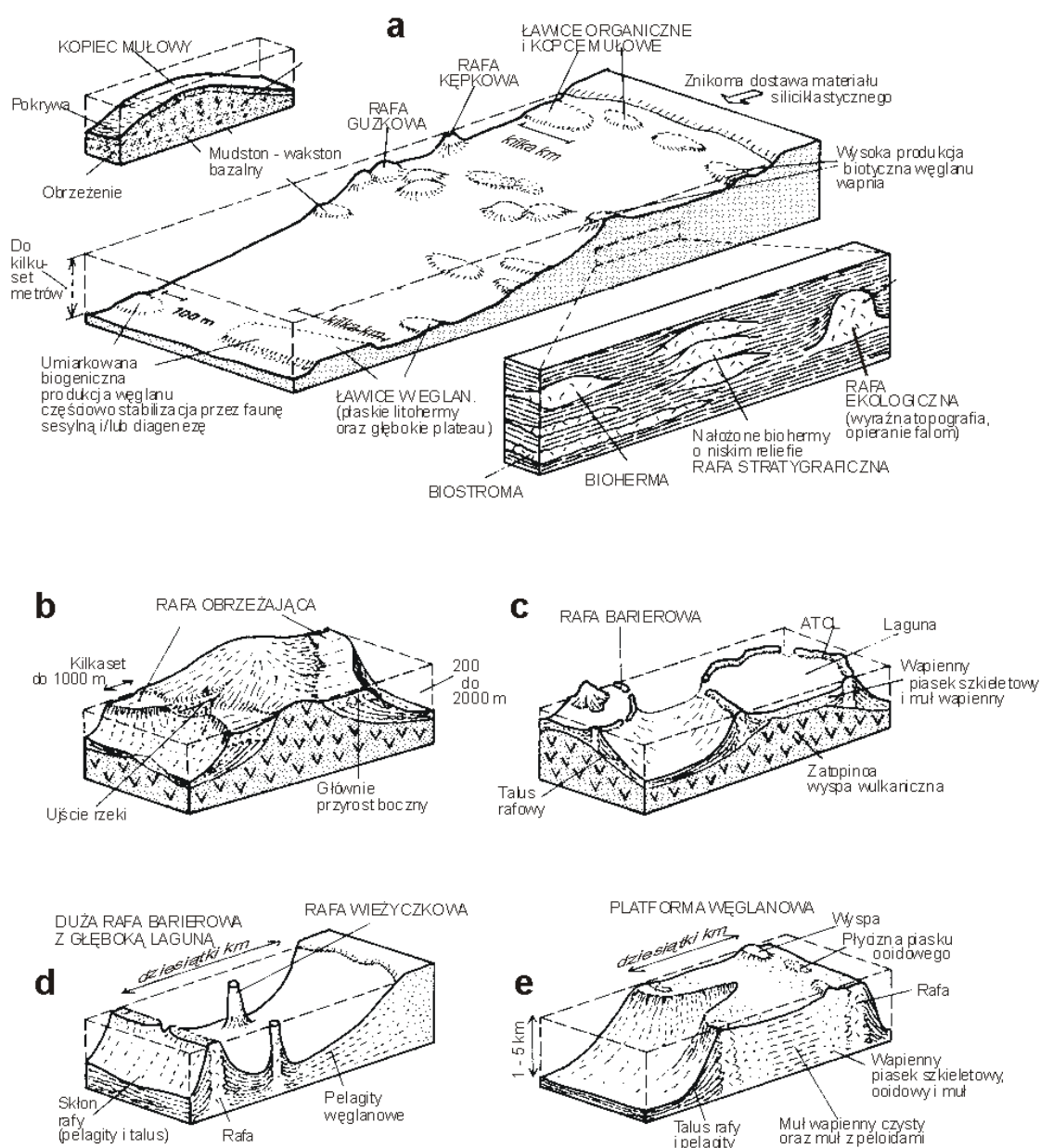
Ryc. 153. Rafy i inne organogeniczne budowle węglanowe, ich rozmieszczenie w morzach współczesnych oraz zapis kopalny (z Einsele 1992)
