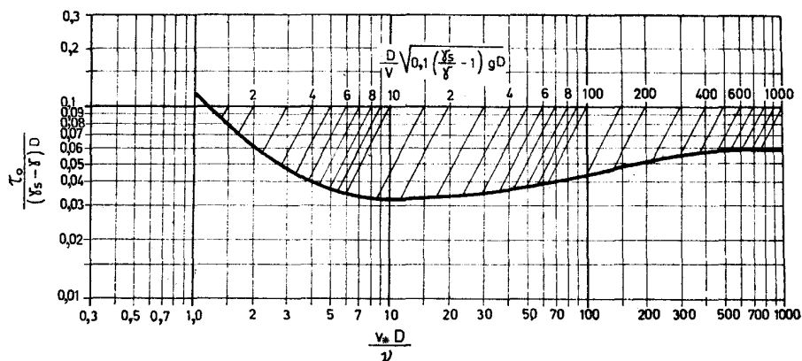
Ryc. 45. Wykres Shieldsa obrazujący warunki progowe ruchu ziaren (z Gradziński et al. 1986)
