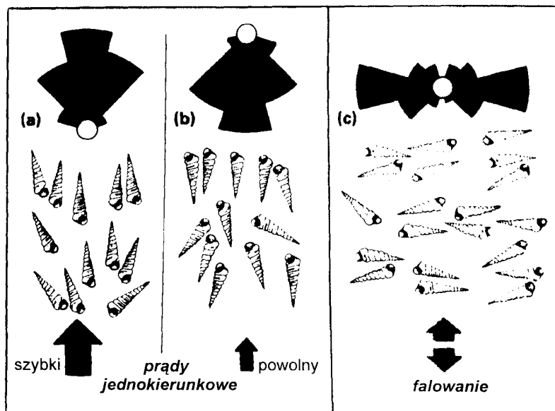
Ryc. 66. Sposoby ułożenia wydłużonych, stożkowych muszli na powierzchni warstwowania. Różne kierunków prądów wskazują kierunek ułożenia wierzchołków muszli (z Lindholm 1987)
