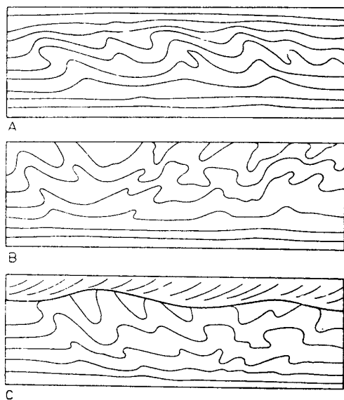
Ryc. 130. Zaburzenia konwolutyjne. A – wygasające w stropie ławicy, B i C – ścięte przez przykrywającą warstwę
