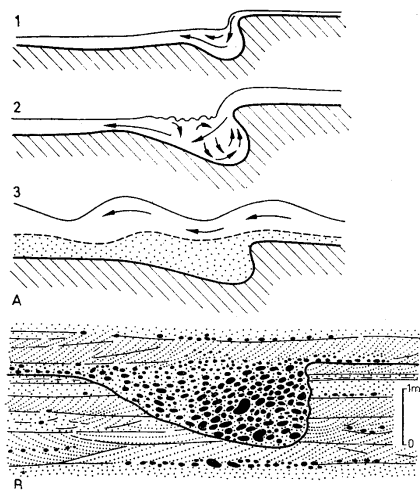
87. Kotły wirowe. A – schemat powstania i zapełniania kotła wirowego według Simons et al., 1965; 1, 2 – erozja podczas niskich stanów wody, 3 – wypełnienie podczas przyboru, B – kopalny kocioł wirowy, formacja Nemeget, Mongolia (według Gradziński 1970), fragmenty mułowców pochodzenia lokalnego zaznaczono kolorem czarnym (z Gradziński et al. 1986)
