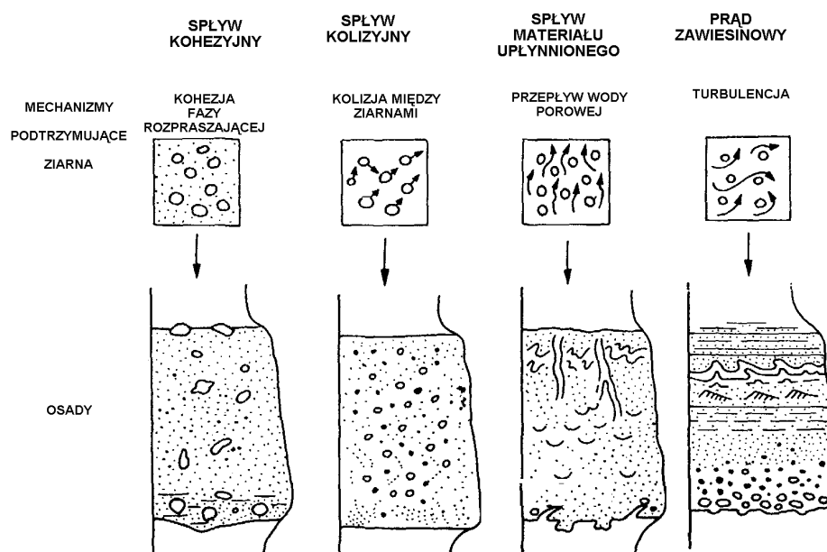
Ryc. 105. Klasyfikacja podwodnych, masowych splywów osadu i ich produktów według Middletona i Hamptona 1973, 1976.
