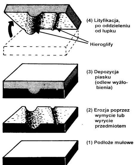
Ryc. 88. Kolejność procesów prowadzących do uformowania hieroglifu
