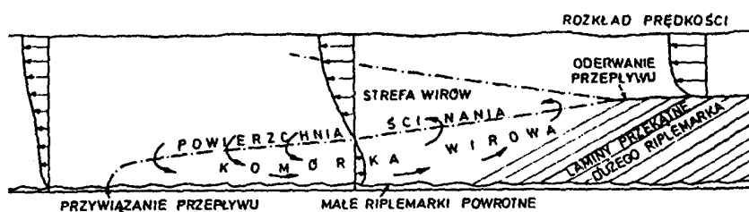
Ryc. 52. Depozycja w obrębie komórki wirowej na zaprawowym stoku riplemarka i na jego przedpolu (z Gradziński et al. 1986)
