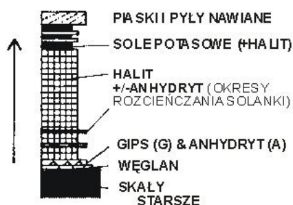
Ryc. 146. Model sedymentacji ewaporatów w basenie o zamkniętym układzie hydrologicznym oraz w panwi solnej (według Einsele, 1992)
