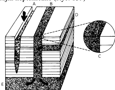
Ryc. 139. Dajka neptuniczna a żyła klastyczna
