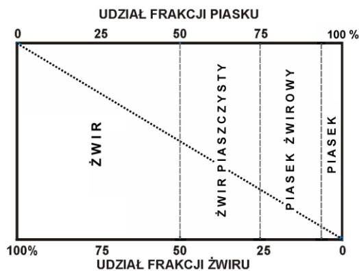
Ryc. 20. Nazwy osadów złożonych z materiału piaszczystego i żwirowego
