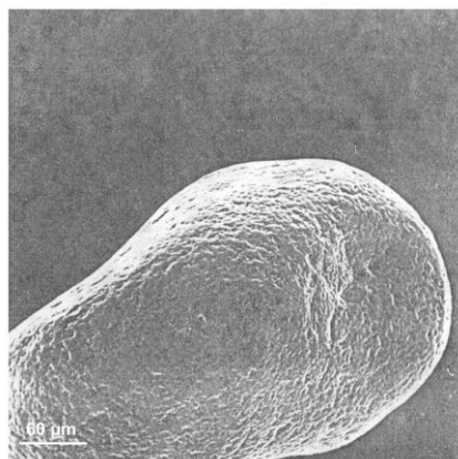
Ryc. 24. Ziarno zaokrąglone, pokryte pochylonymi płytkami. Współczesny piasek wydmowy; Sahara
