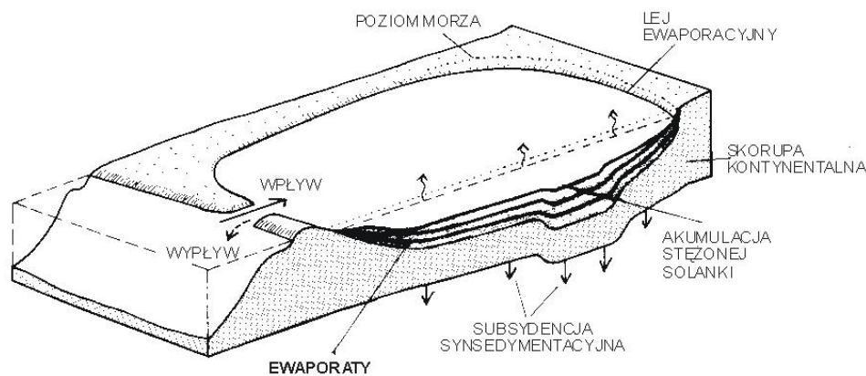
Ryc. 149. Model sedymentacji ewaporatów w basenie zasilanym przez przegrodę, podlegającym subsydencji (według Einsele 1992)
