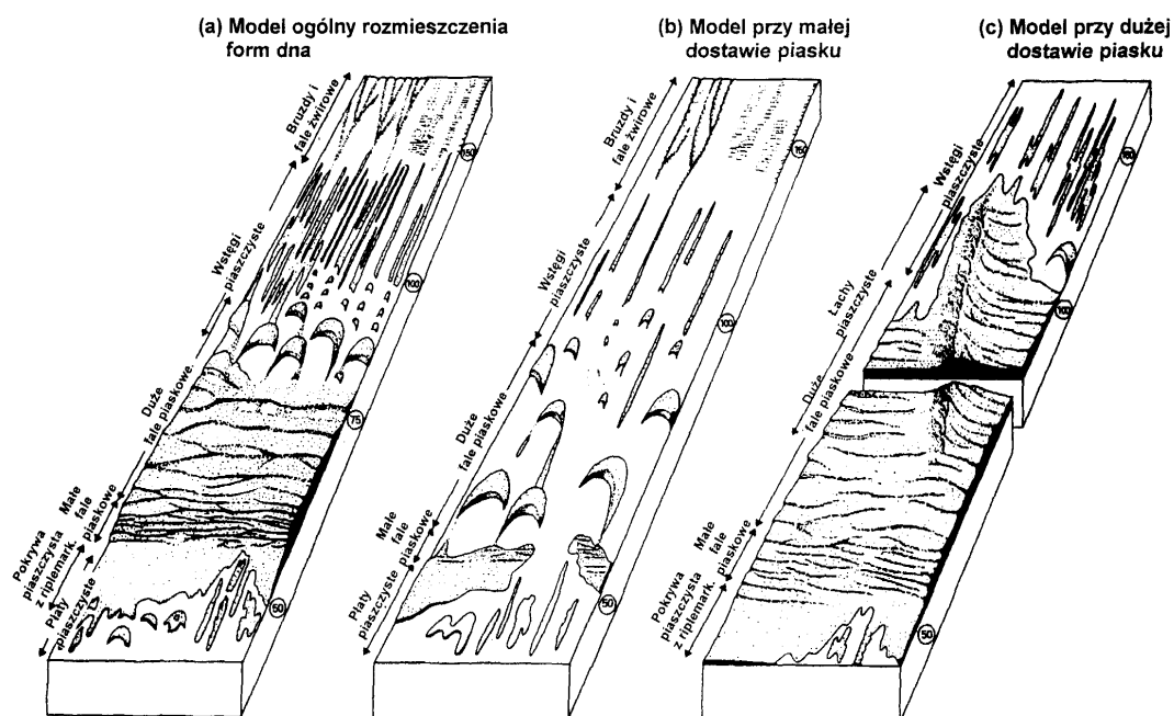
Ryc. 83. Formy osadu kształtowane długookresowo przez pływy i ich następstwo na pełnej trasie transportu osadu. Liczby oznaczają prędkości najsilniejszego, przypowierzchniowego prądu syzygiowego w cm/s (wg Belderson et al. 1982)
