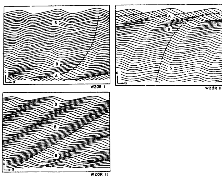
Ryc. 60. Wzory riplemarków wstępujących (z Gradziński et al. 1986)
