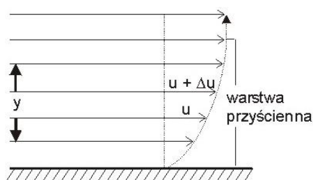
Ryc. 36. Ilustracja wyrazu warstwy przyściennej
