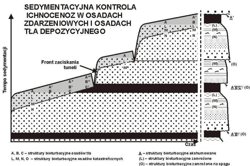
Ryc. 168. Produkcja i fosylizacja struktur bioturbacyjnych w osadach zdarzeniowych i osadach tła depozycyjnego (według Leszczyński 1993)
