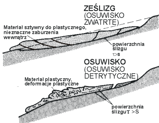
Ryc. 112. Zasadnicze cechy charakterystyczne ześlizgów i osuwisk
