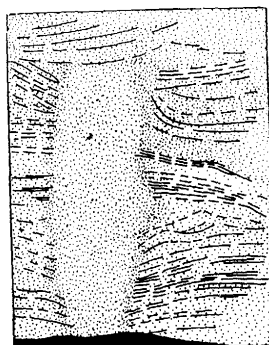
Ryc. 138. Kanał uciezkowy (wg Gradziński et al. 1986)
