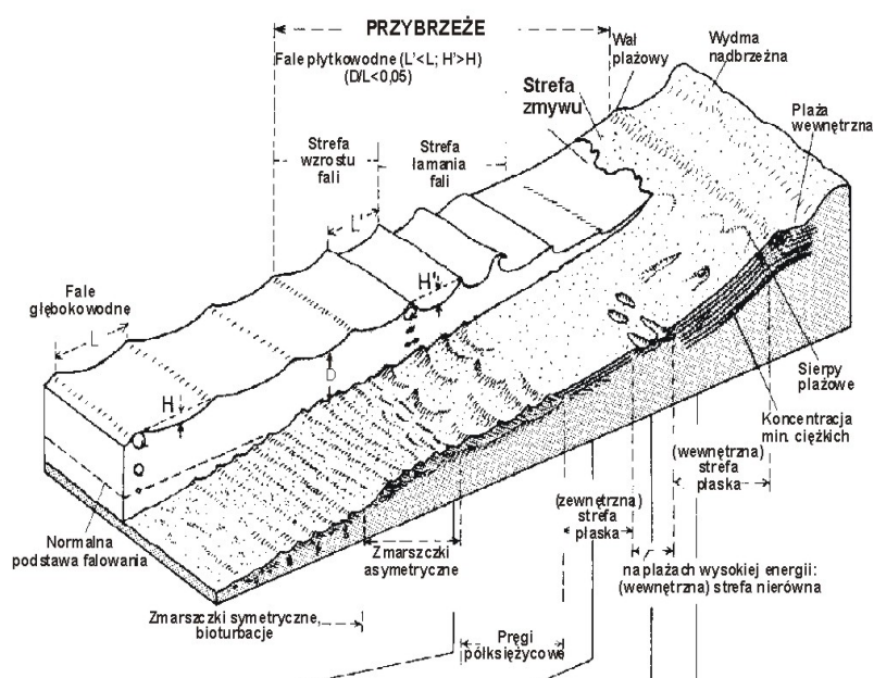
Ryc. 73. Formy dna na wybrzeżu bezrewowym, zależnie od dynamiki wody: stan w warunkach intensywnego falowania (z Einsele 1992).
