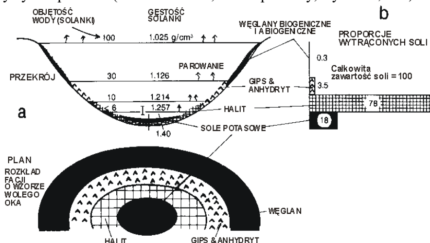
Ryc. 146. Model sedymentacji ewaporatów w basenie o zamkniętym układzie hydrologicznym oraz w panwi solnej (według Einsele, 1992)
