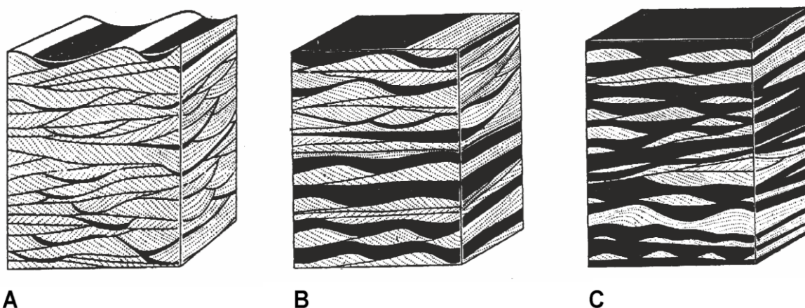
Ryc. 67. Warstwowanie smużyste (A), faliste (B) i soczewkowe (C) (z Gradziński et al. 1986)
