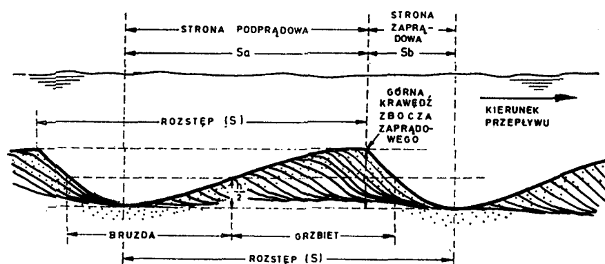
Ryc. 49. Budowa zmarszczka (riplemarka małego), pręgi (riplemarka dużego) w przekroju (z Gradziński et al. 1975)
