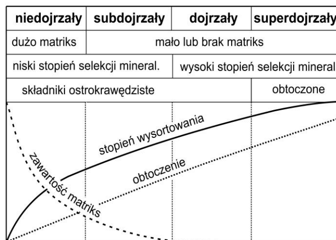
Ryc. 30. Stopień dojrzałości materiału osadowego (osadu) wg Folka (1979)
