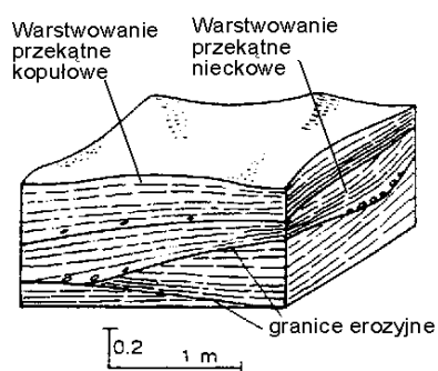
Ryc. 77. Warstwowanie przekątne kopułowe-nieckowe (wg Einsele 1992)
