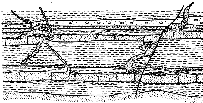
Ryc. 134. Żyły piaskowcowe w utworach fliszowych; Karpaty (z Gradziński et al. 1986)
