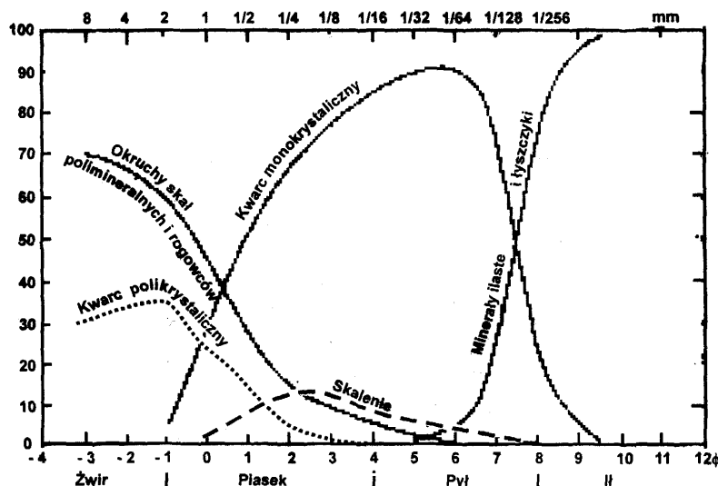
Ryc. 7. Wielkość ziarna a skład mineralny osadu
