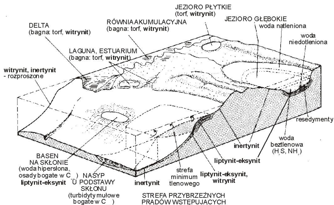
Ryc. 156. Środowiska wzmózonej akumulacji materii organicznej i jej rodzaje (macerały) według Einsele, 1992
