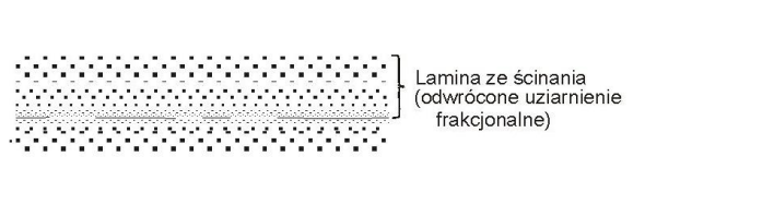
Ryc. 42. Budowa laminy ze ścinania w przekroju
