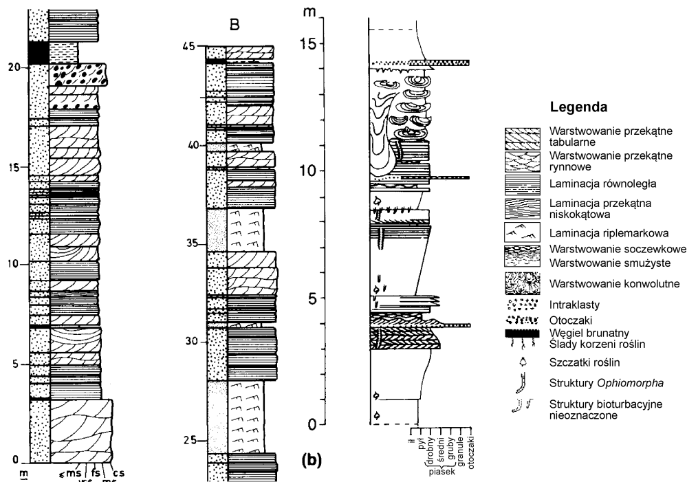
Ryc. 4. Przykłady profili sedimentologicznych
