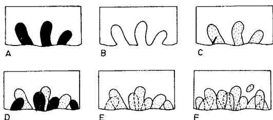
Ryc. 158. Stadia powstawania osłony mikrytovej na ziarnie wapiennym (według Bathurst, 1966, zmienione przez Gradziński et al. , 1986) A – glony drążą w elemencie szkieletowym kanaliki, B – puste wydrążenia po wymarłych i rozłożonych glonach, C – wydrążenia wypełnione mikrytem, D – powtórna kolonizacja szkieletu przez glony, E – wypełnianie mikrytem nowych wydrążeń, F – powstanie ciągłej powłoki mikrytovej
