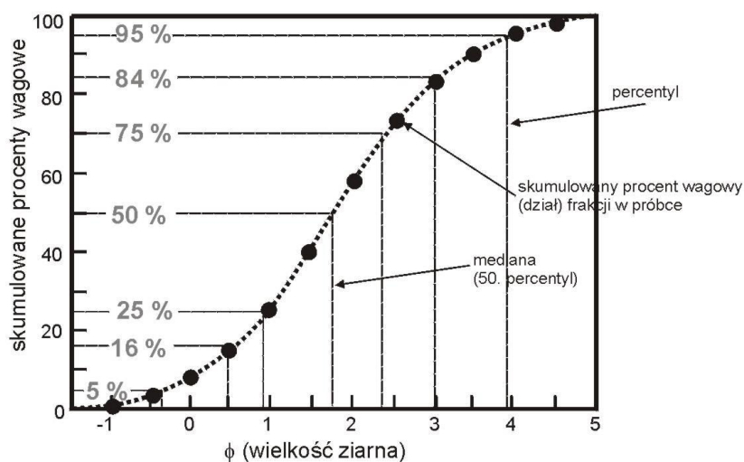
Ryc. 13. Sporządzenie krzywej kumulacyjnej, określanie percentyli i mediany. Czarne punkty na krzywej kumulacyjnej (podstawa wykreślenia krzywej kumulacyjnej), to skumulowane procenty wagowe poszczególnych frakcji wydzielonych w analizie rozkładu wielkości ziarna w próbce (patrz Ryc. 8)
