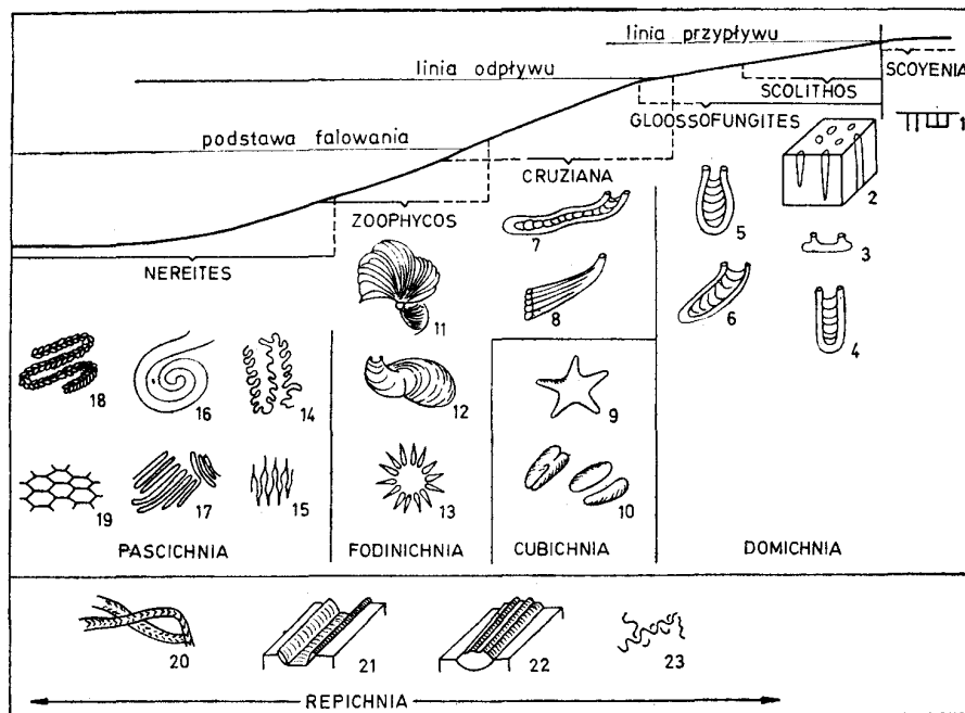
Ryc. 165. Batymetryczne rozmieszczenie zespołów skamieniałości śladowych (ichnofacji) według Seilachera.
