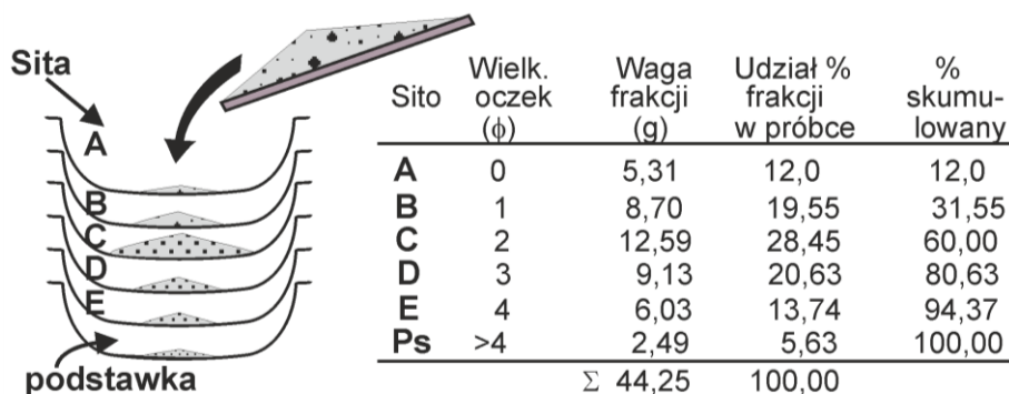
Ryc. 8. Zasadnicze kroki sitowej analizy granulometrycznej
