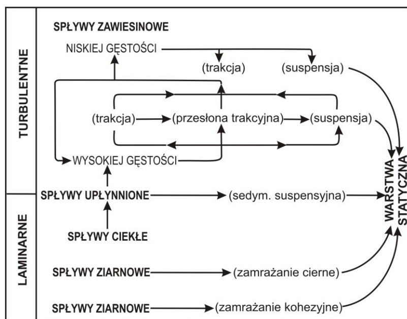
Ryc. 108. Podstawowe sposoby depozycji z grawitacyjnych spływów osadu (według Lowe 1982)
