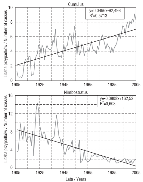
Ryc. 4. Przebieg wieloletni częstości chmury Cumulus i Nimbostratus w Krakowie (1906-2005)
