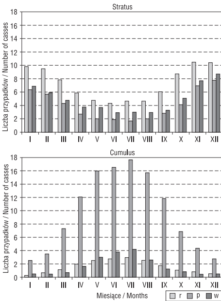
Ryc. 3. Przebieg roczny częstości chmury Stratus i Cumulus w Krakowie (1906-2005) w terminach klimatologicznych: r – rano, p – południe, w – wieczór
