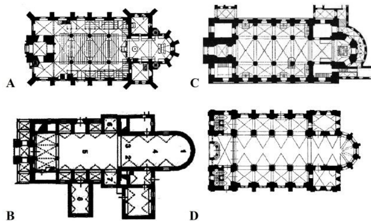
9 Floor plans of A) Marienkirche, Wolfenbüttel | B) Holy Trinity Church, Klagenfurt | C) Court Church, Neuburg an der Donau | D) St Salvator's Church, Prague (reprod. from: A) Gustav von Bezold, Die Baukunst der Renaissance in Deutschland, Holland, Belgien und Dänemark , Leipzig 1908, 129; B) https://www.kath-kirche-kaernten.at/pfarren/detail/C3074/ein_fuehrer_durch_die_domkirche [accessed February 12, 2021]; C) and D) Praha 1437–1610 , ed. Pavel Kalina and Jiří Kotatko, Prague 2011, 163)
