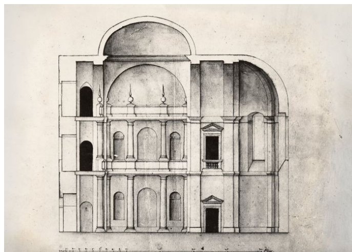
14 Valentin von Saebisch, Cross-section design of the Carolath Castle chapel, 1616 (reprod. from: Günther Grundmann, Der evangelische Kirchenbau in Schlesien , Frankfurt am Main 1970, 115)
