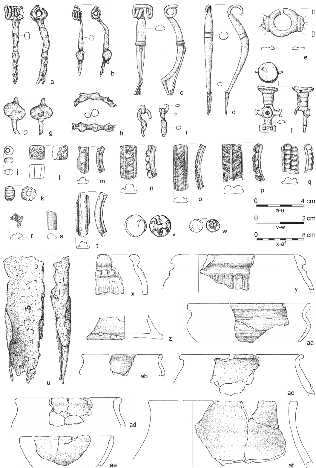
Ryc. 4. Podlęża, stan. 17. Wybór materiału z obiektów i nawarstwień kulturowych: a-b, g-i, u – żelazo; c-e – brąz; f – brąz i żelazo; j-t – szkło; v – srebro; w – złoto; x-aa – ceramika wykonana na kole; ab-af – ceramika lepiona ręcznie.
