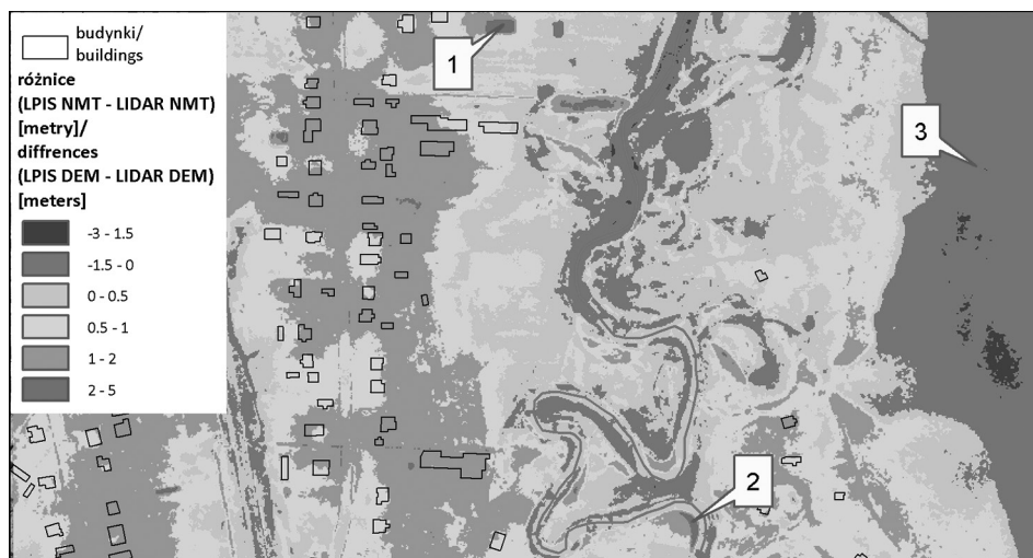
Ryc. 1. Różnice w modelach terenu na obszarze analizy, 1 – wykoppy, 2 – działalność erozyjna rzeki, 3 – las
